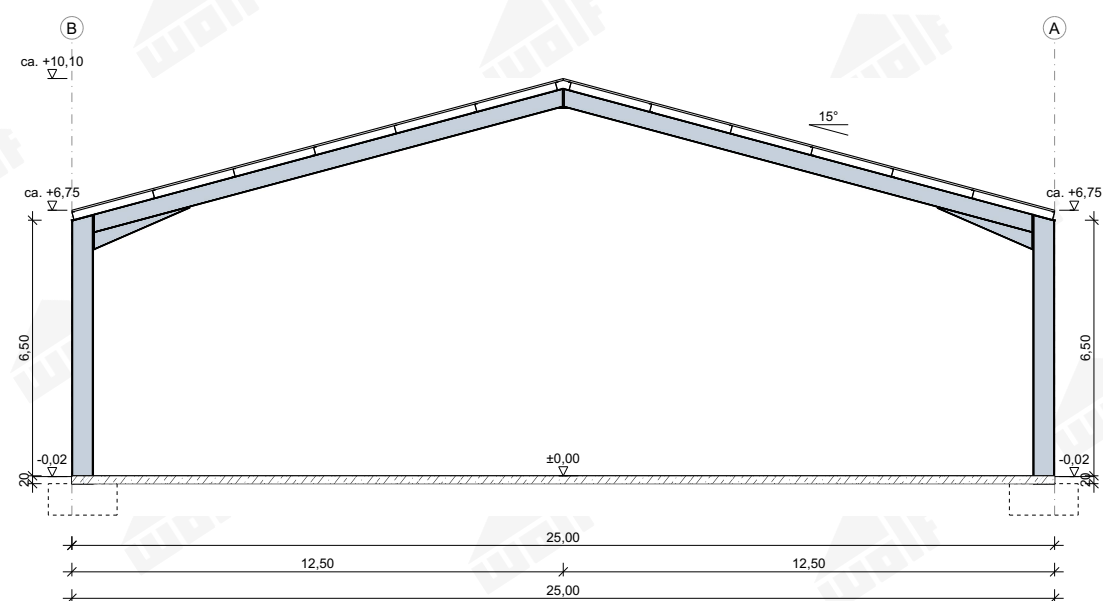
Schnitt A-A
